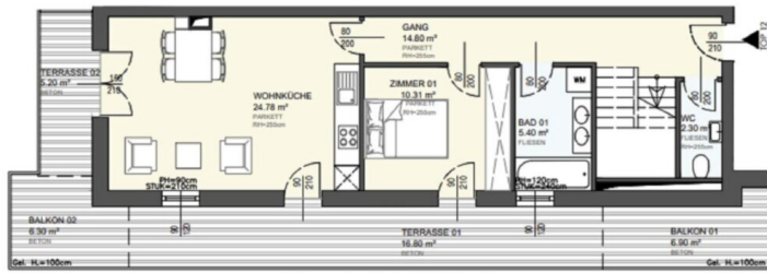
1. DACHGESCHOSS
