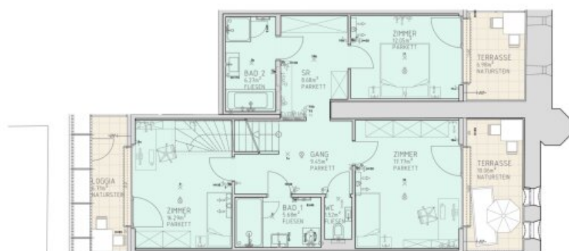
1.DACHGESCHOSS M 1:75
