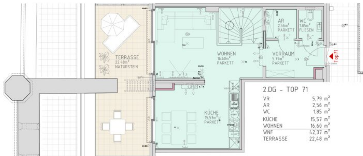
2.DACHGESCHOSS M 1:50
