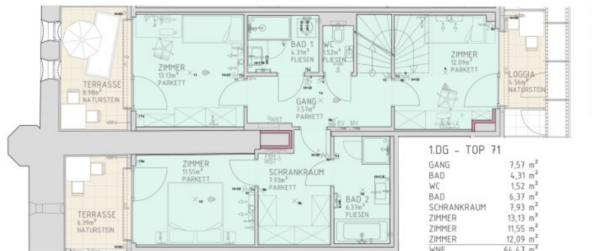
1.DACHGESCHOSS M 1:50
