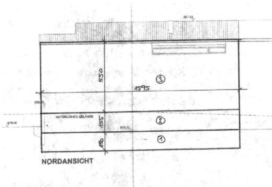
Nordansicht
