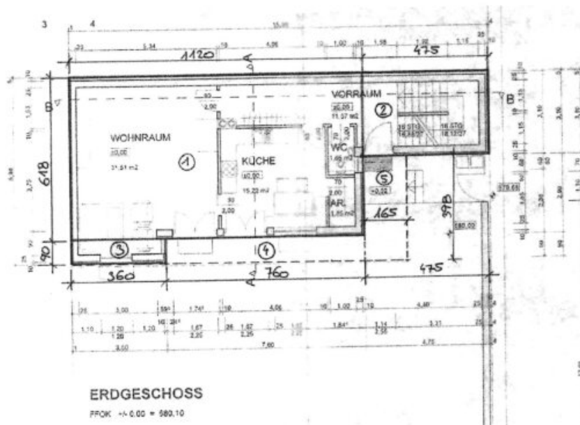
Erdgeschoß
