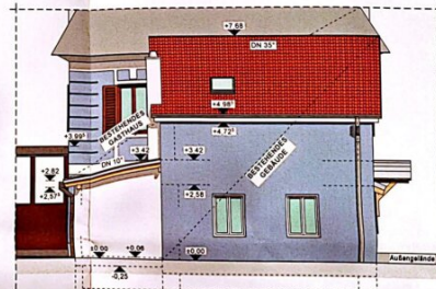
WESTANSICHT
