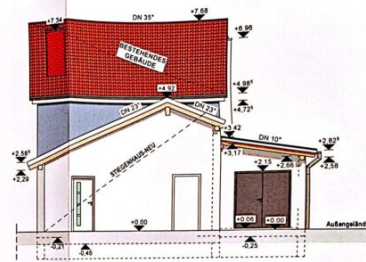
OSTANSICHT
