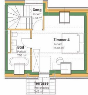
Dachgeschoss
