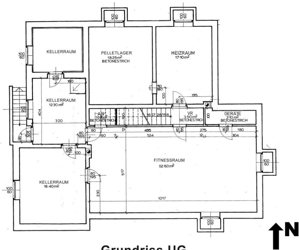
Grundriss UG
