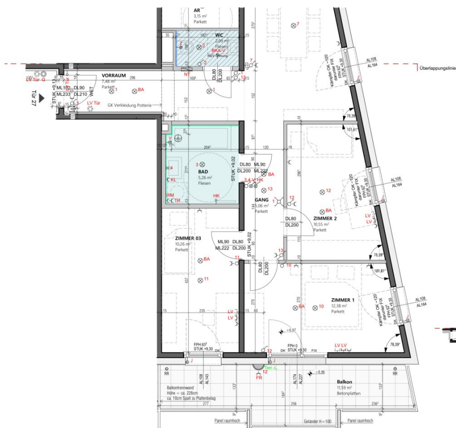
Übersichtsplan
