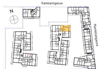
ÜBERSICHTSPLAN- 2.OG
