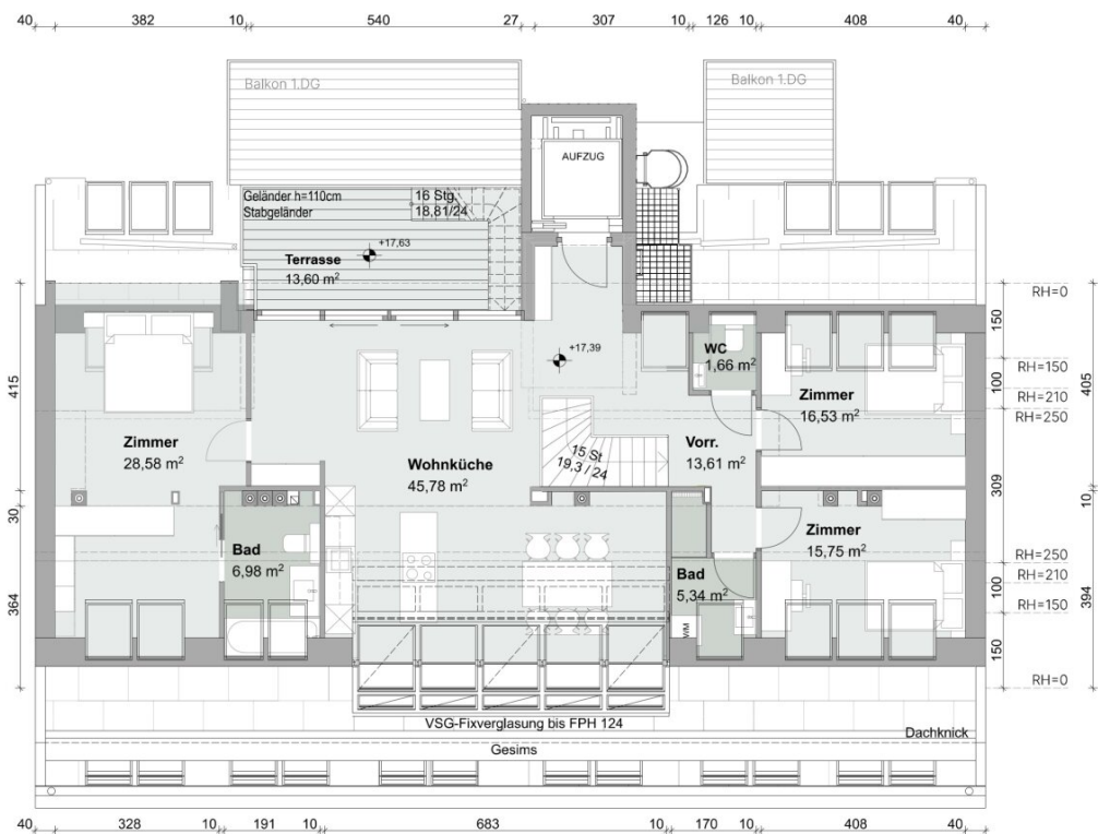
Dachterrasse
