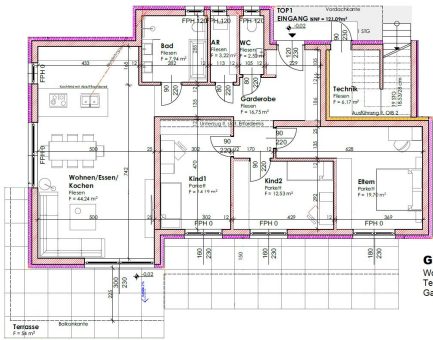
Grundriss Top 1 Wohnfläche 121m 2 Terrasse 54m 2 Garten 198m 2
