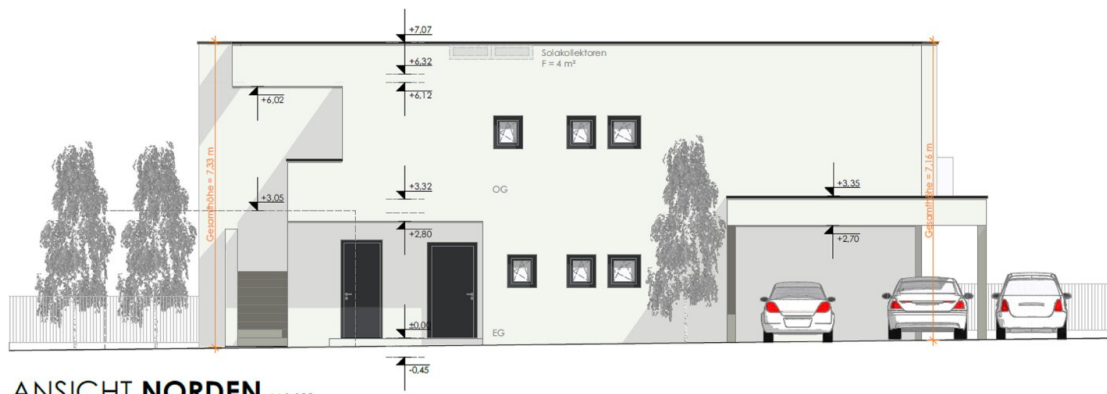
ANSICHT NORDEN M 1:100
