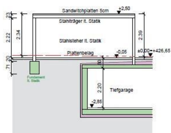
SCHNITT Nebenanlage
