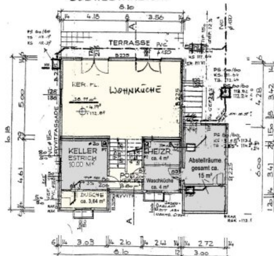
KELLERGECHOSS
