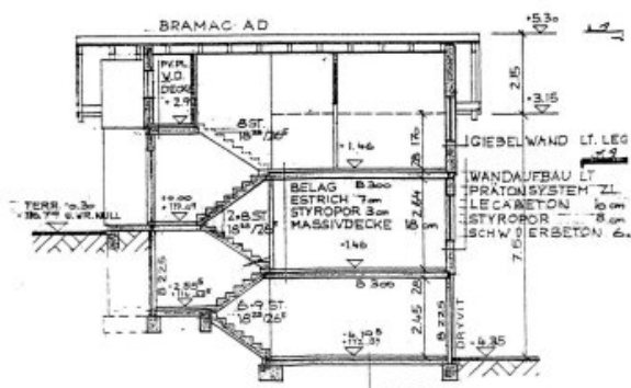
SCHNITT
