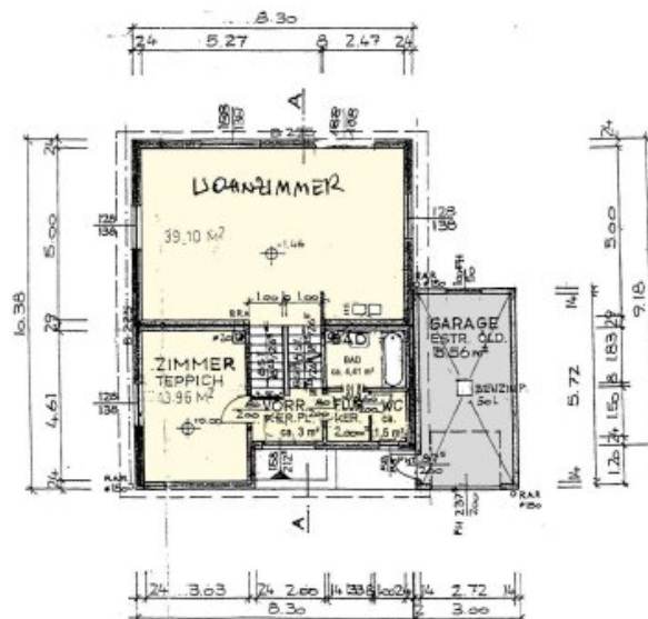
ERDGESCHOSS
