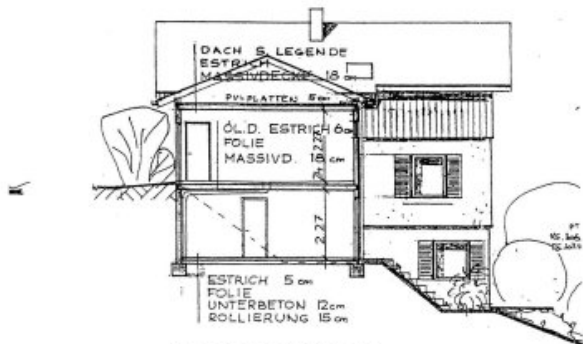
NORDOSTANSICHT
