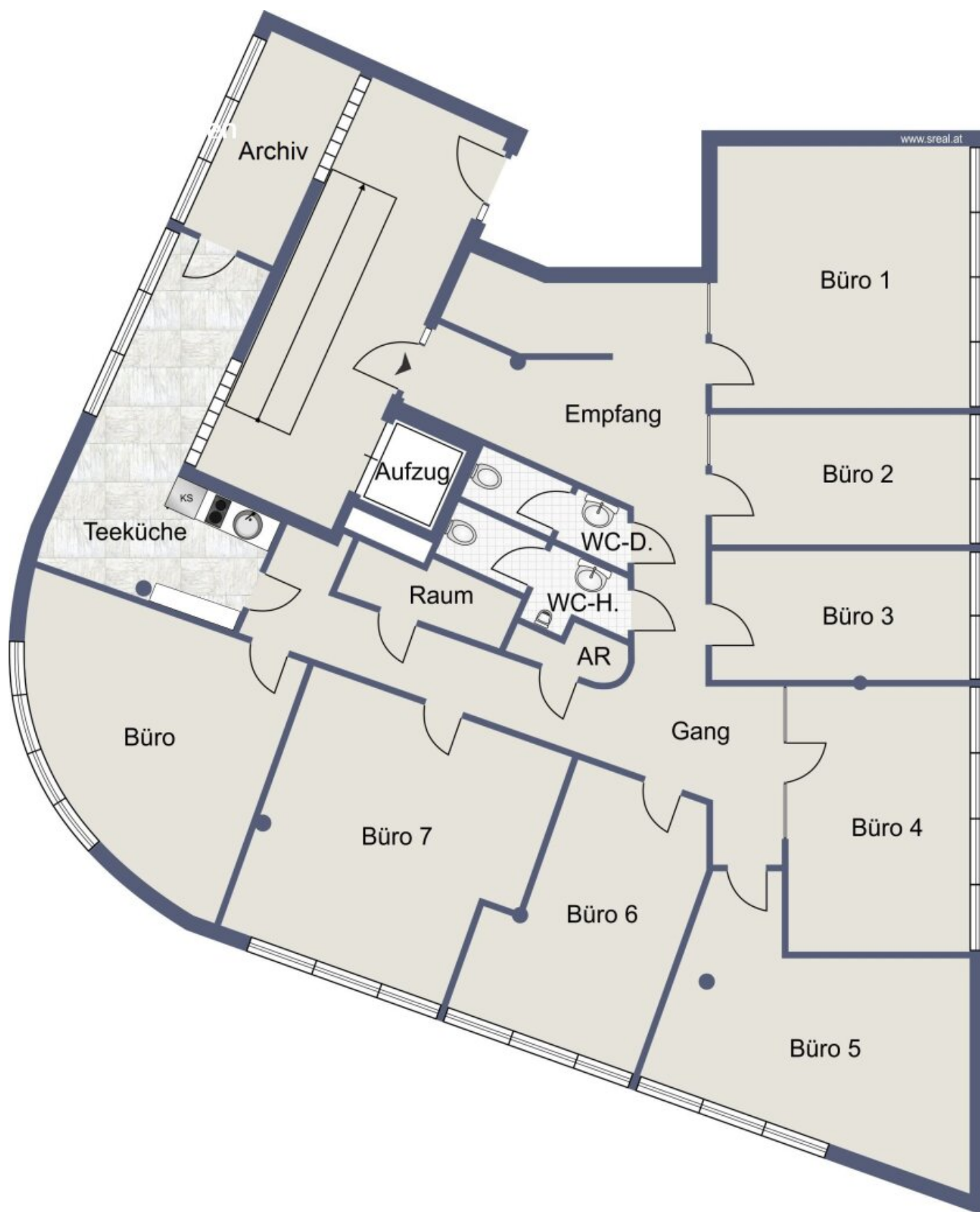
Skizze Obergeschoss 2
