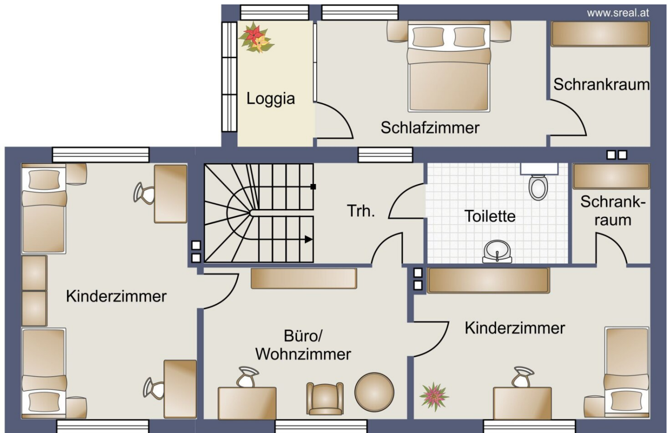
Skizze 1. Obergeschoss
