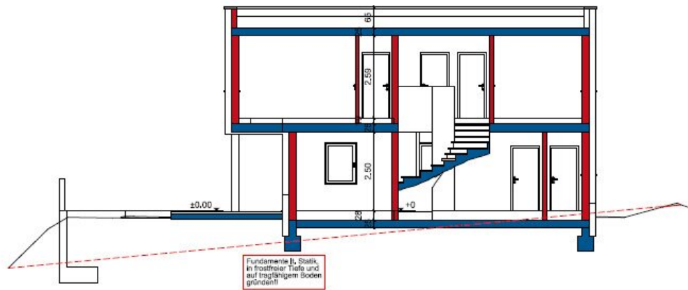
SCHNITT A-A
