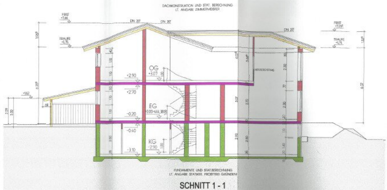
WOHNHAUS
