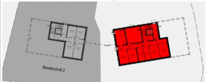
Übersicht Grundriss Kellergeschoss M500
