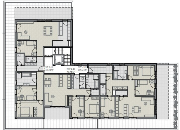
Dachgeschoß
