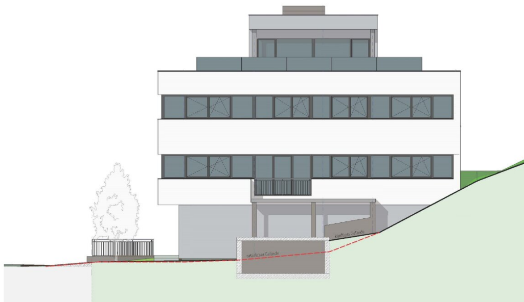
Seitenansicht Ost
