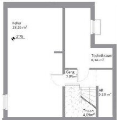
KELLERGECHOSS NF 47,84m 2
