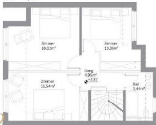
DZWERTSGESCHOSS WNF 58,01m 2
