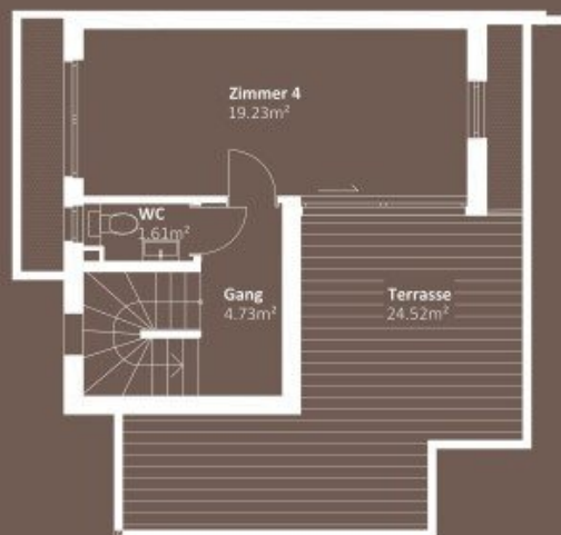
DACHGESCHOSS WNF 25,57m²
