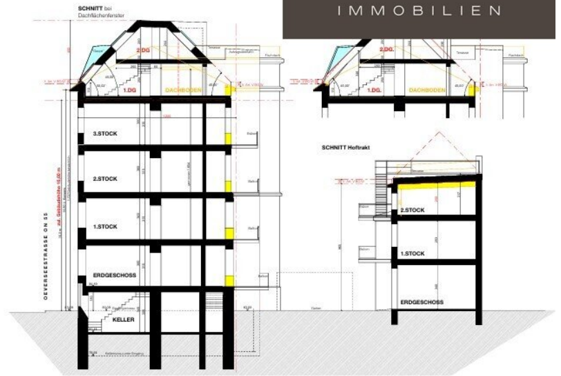
SCHNITT AA
