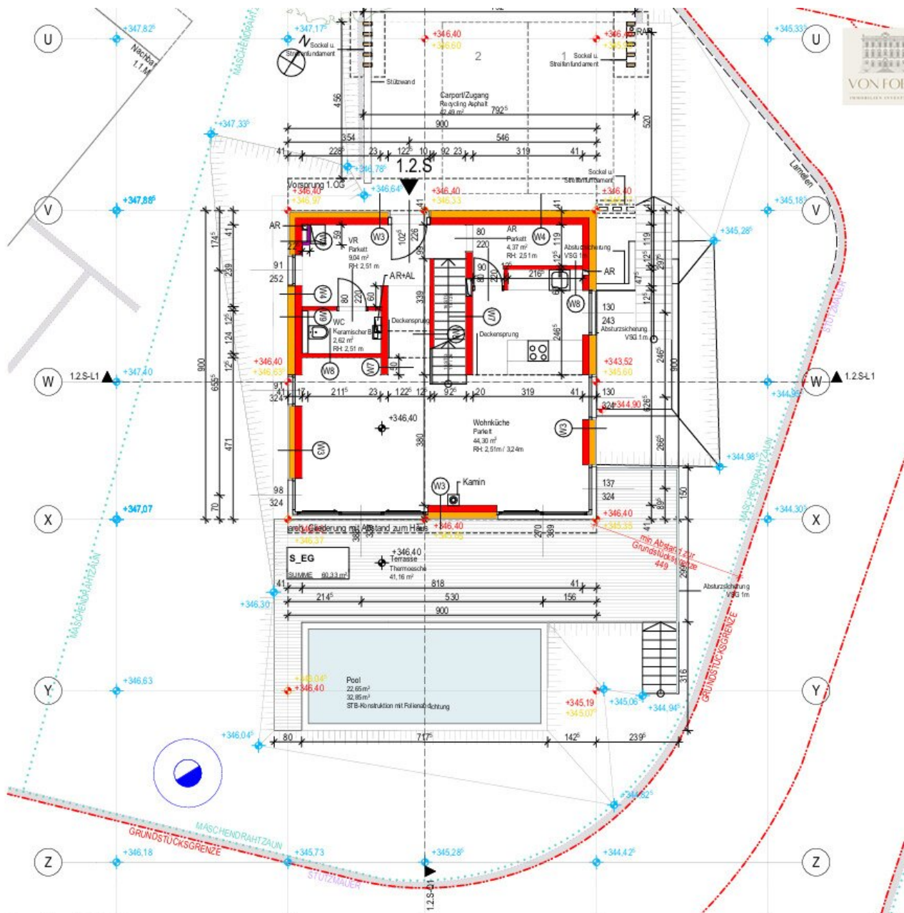
Grundriss 1.2.S-EG
