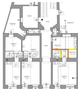
GRUNDRISS EG
