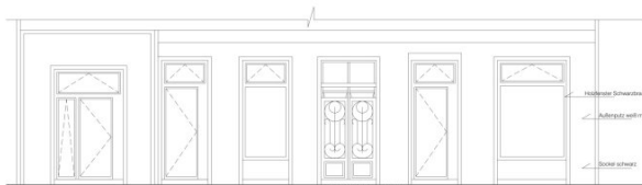
ANSICHT EG 1-50
