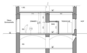
SCHNITT 1-1
