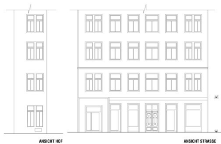
ANSICHT HOF
