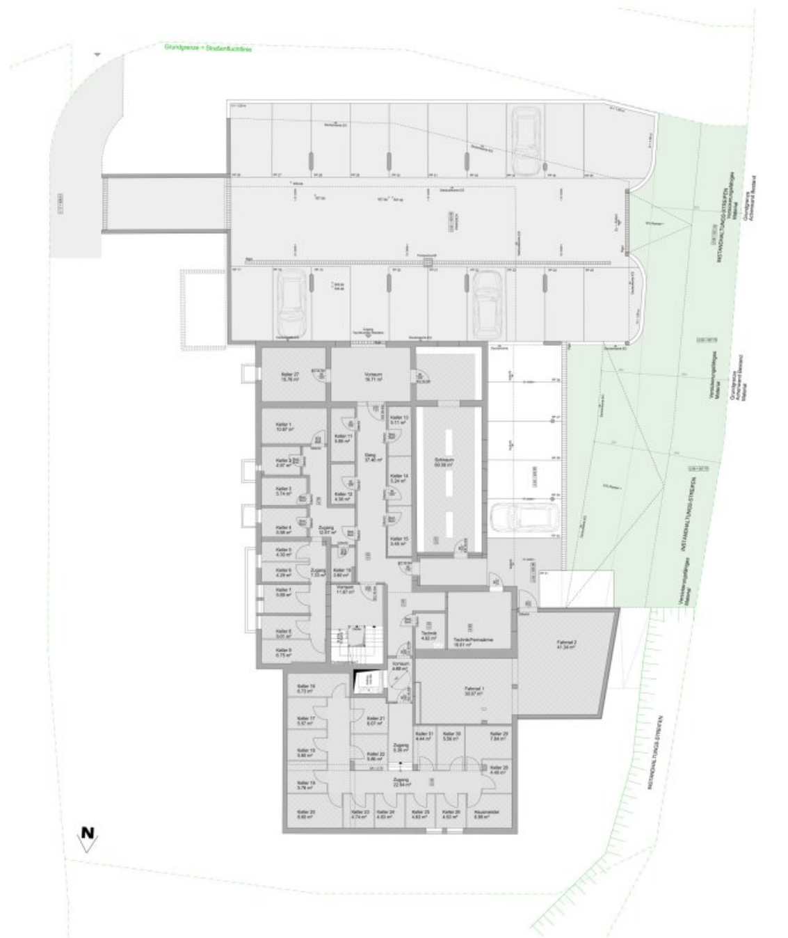
Grundriss Untergeschoss
