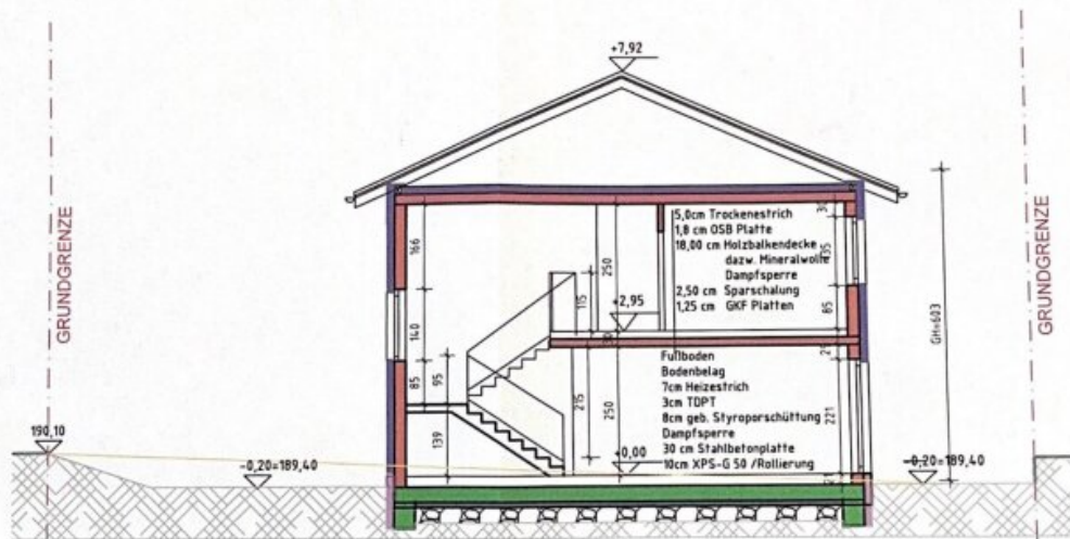
SNITT B-B
