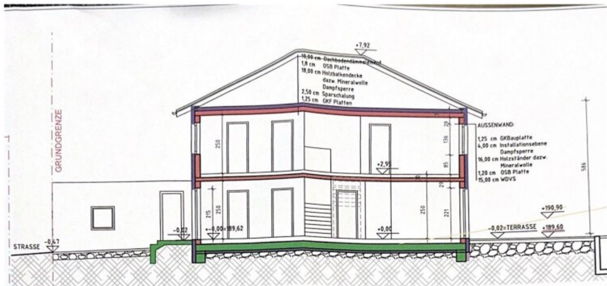
SNITT A-A
