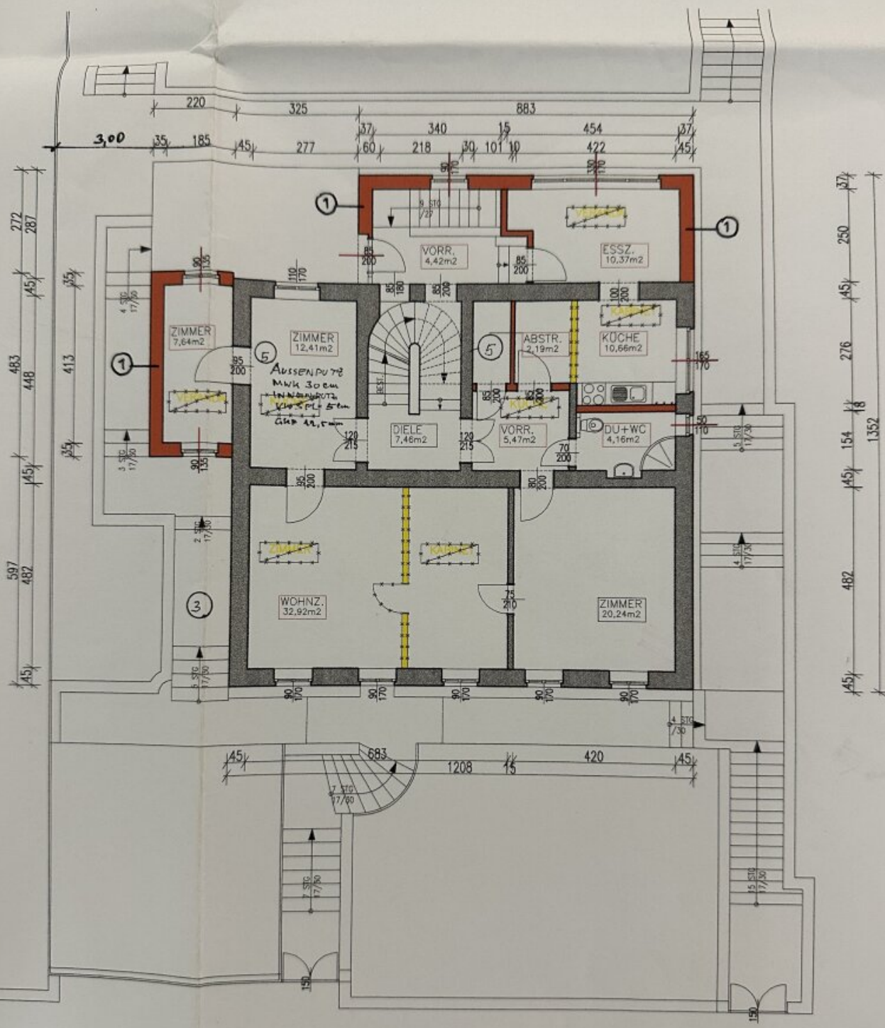
ERDGESCHOSS
