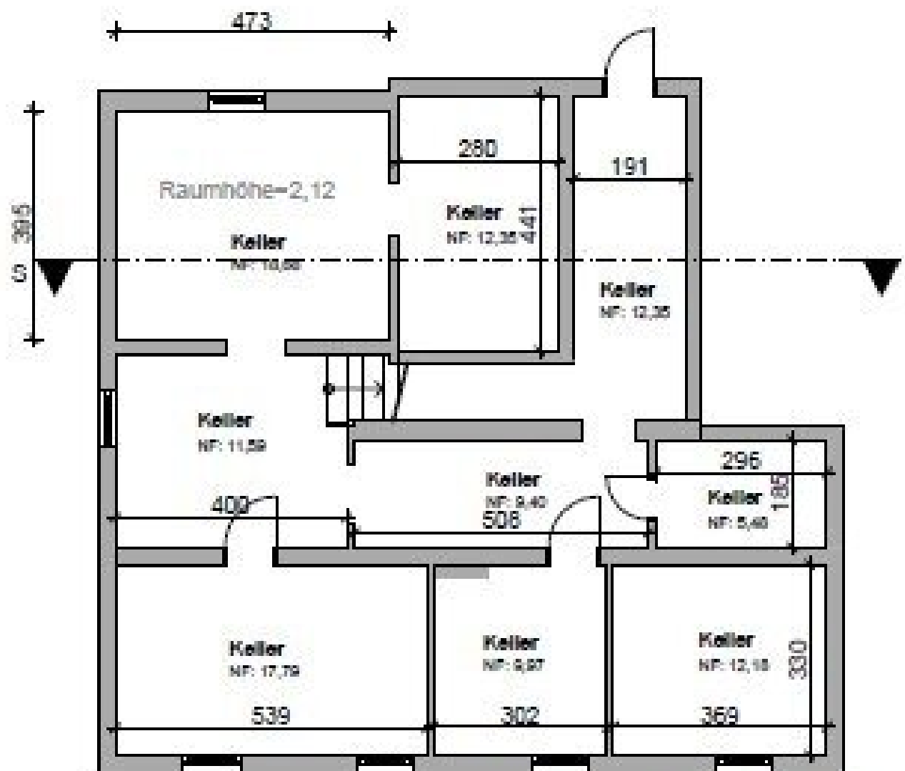
KELLERGECHOSS
