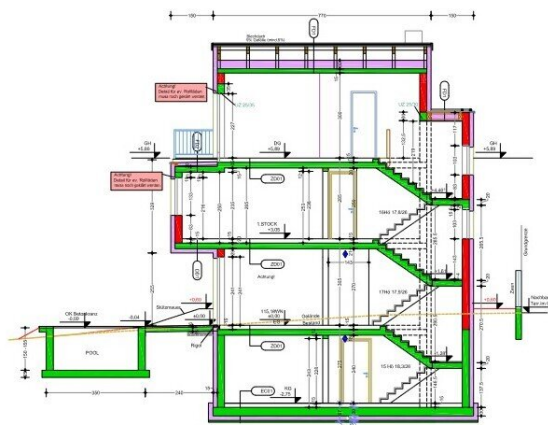
SCHNITT 2-2
