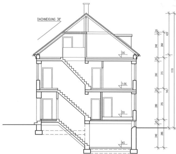
SCHNITT A-A
