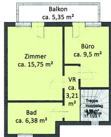
Obergeschoß
