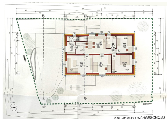
GRUNDRISS DACHGESCHOSS
