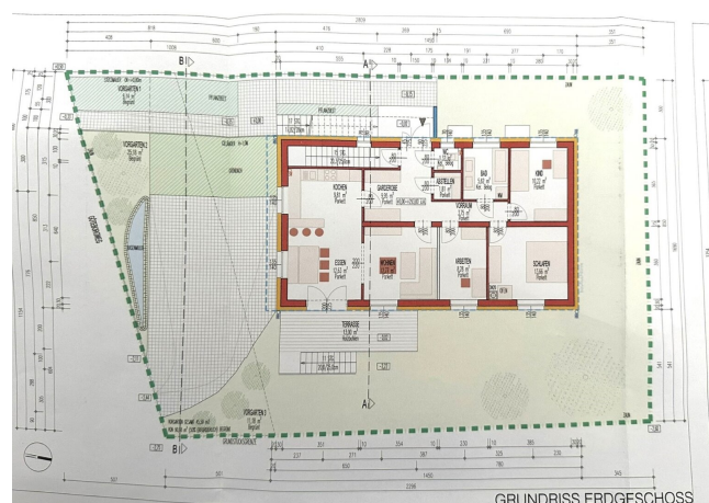
GRUNDRISS ERDGESCHOSS
