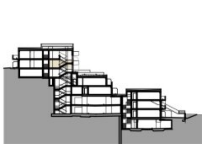
SCHNITT BK 02+04
