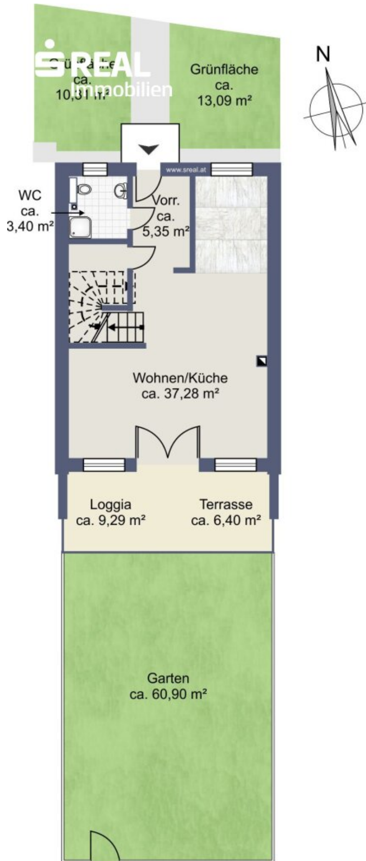
Skizze Erdgeschoss
