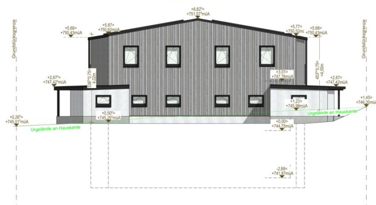
ANSICHT NORD
