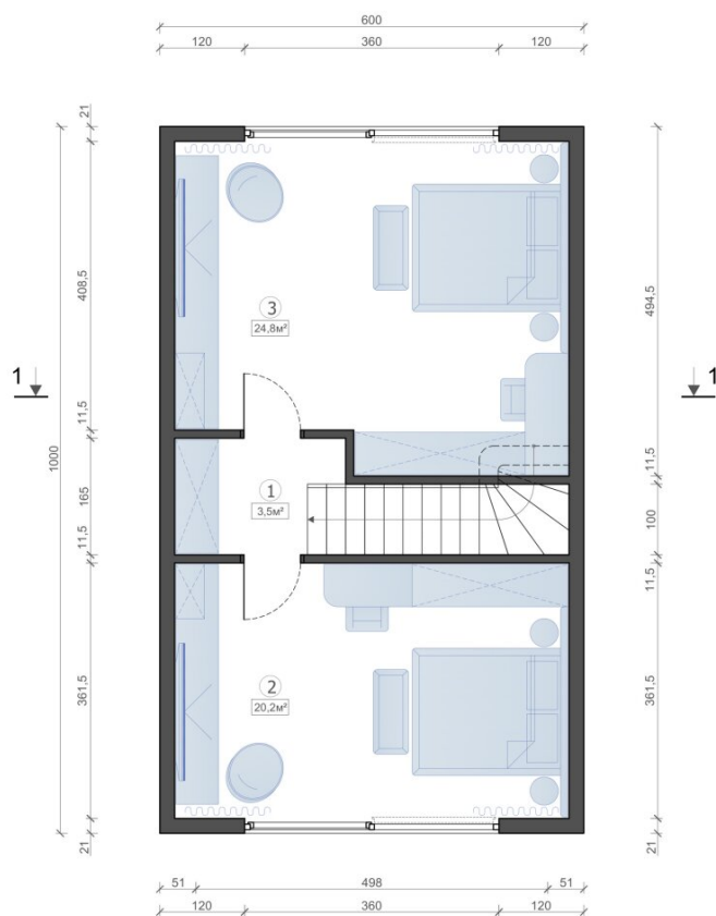
Obergeschoss. M 1:50 (A-3)
