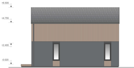
Fassade 4. M 1:50 (A-3)
