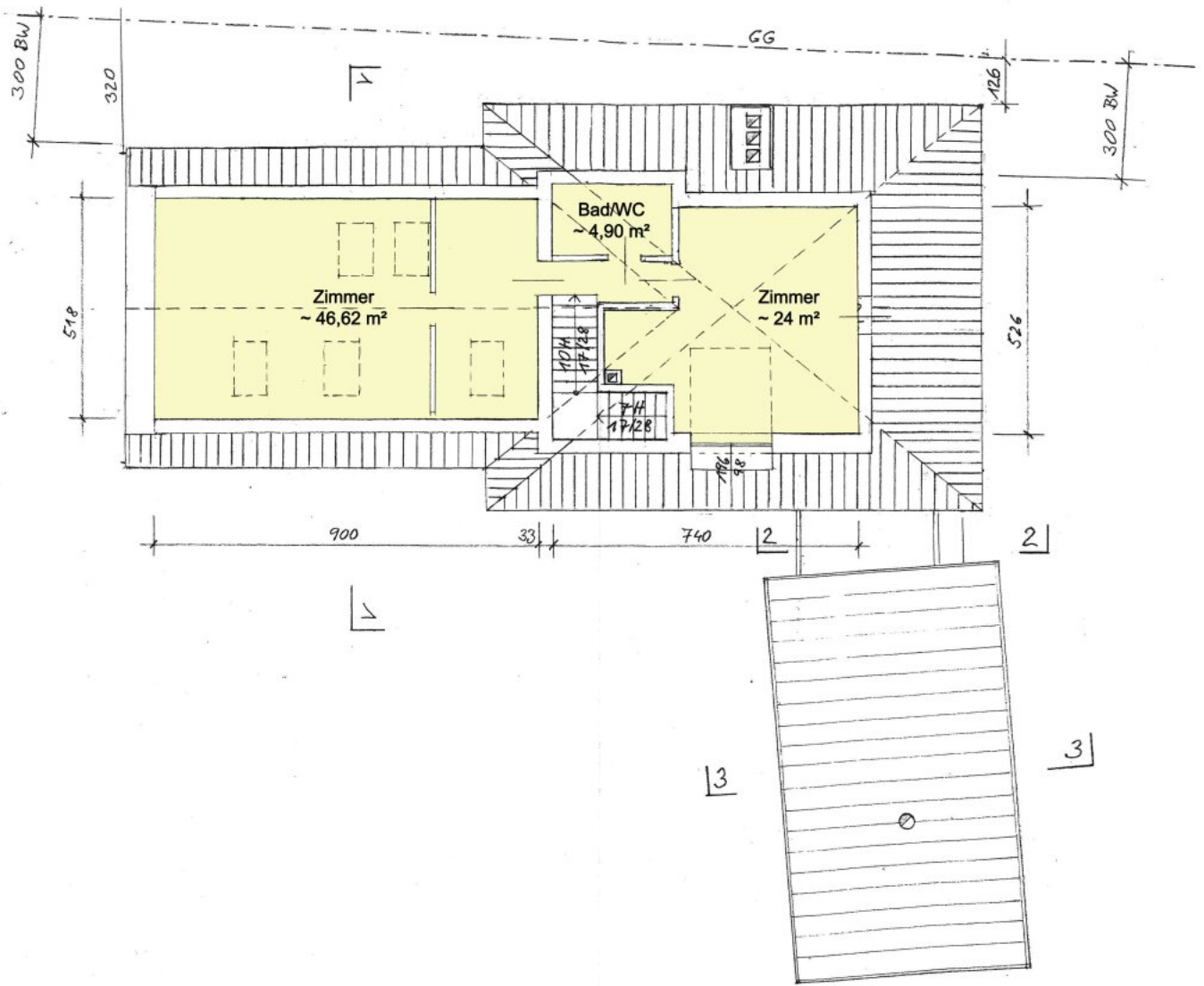
DACHGESCHOSS + DACHDRAUFSICHT
