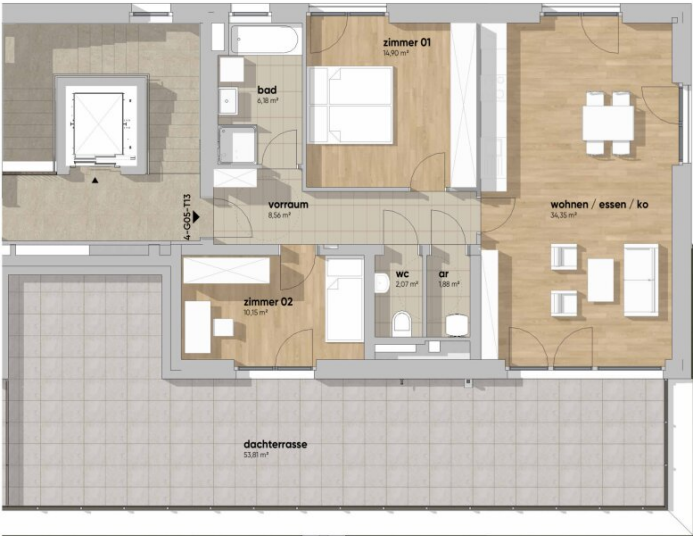
grundriss M 1:75
