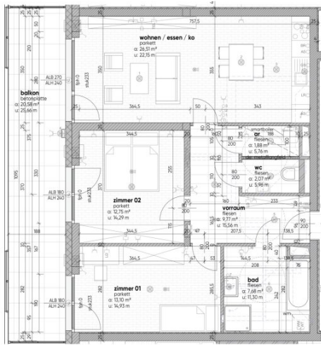
grundriss mit technik M 1:75
