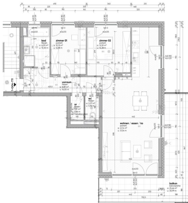
grundriss mit technik M1:75
