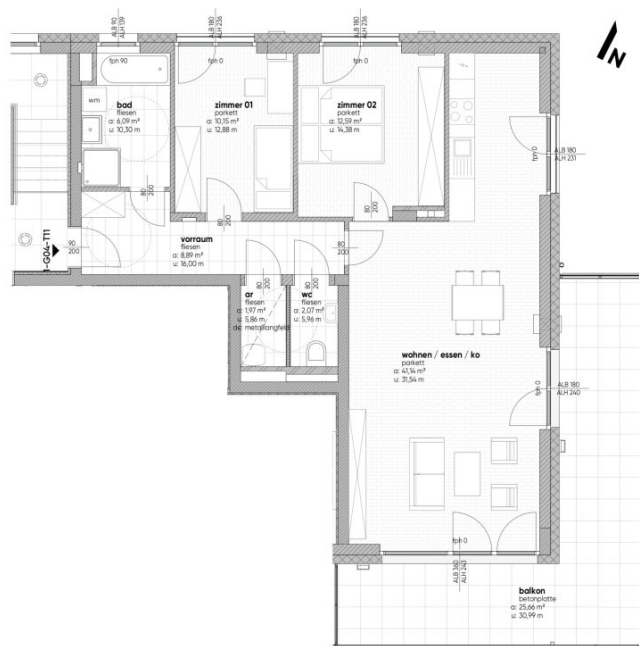
grundriss M 1:75
