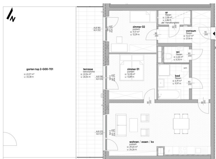
grundriss M1:75
