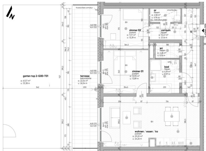
grundriss mit technik M1:75
