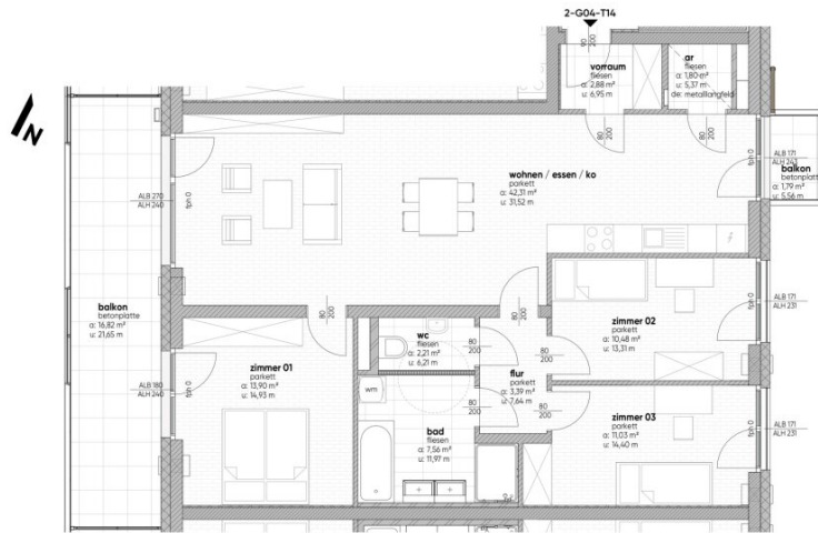
grundriss M1:75
