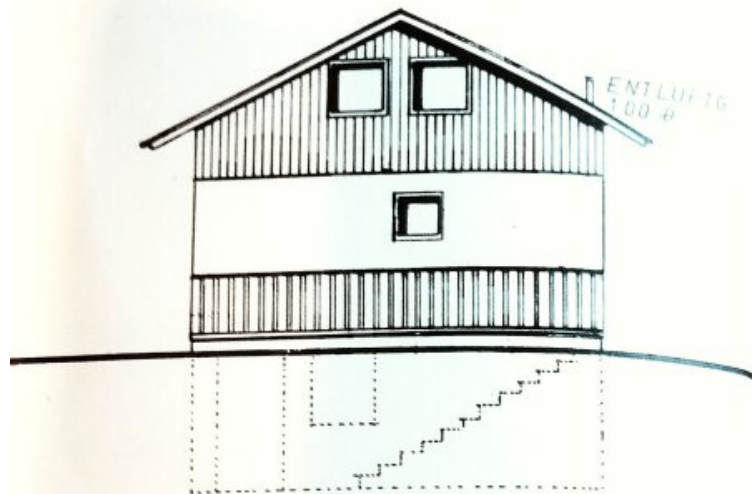
O-ANSICHT
