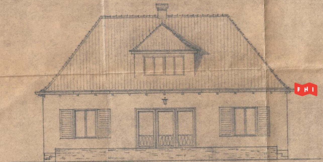
LANGSANSICHT, + SÜD-WEST +
