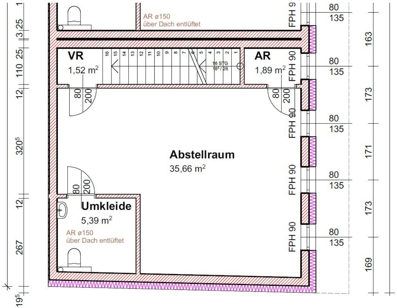
GRUNDRISS OBERGESCHOSS
