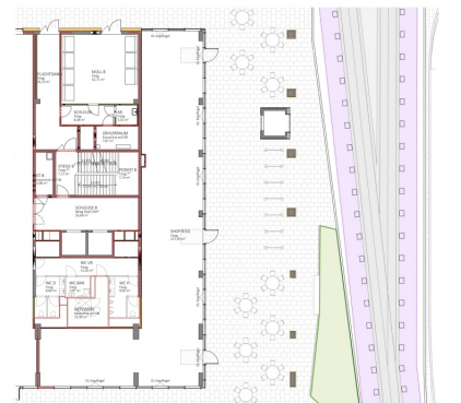
0 m 5 m 10 m Fläche Shop B ohne Kern 217,95m 2
