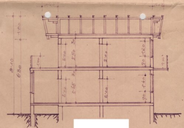
SCHEIT A-B
