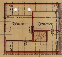
Dachgeschloß
