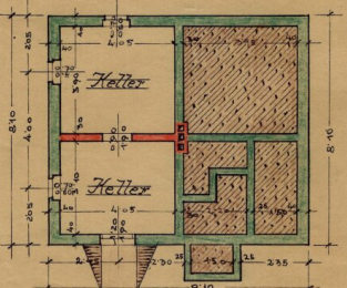
Kellergerüst
