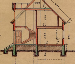
Schnitt A-B
