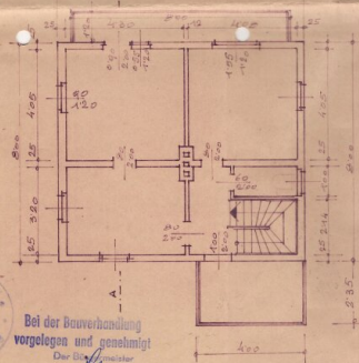
OBERGESCHOSS
