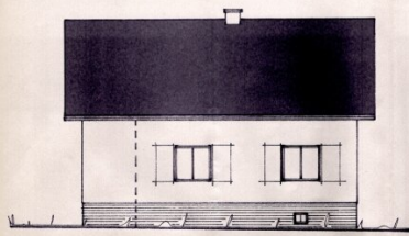
SÜD - WEST
