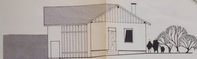
NORD-OST ANSICHT M 1:100
