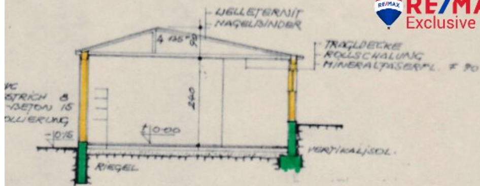
SCHNITT 1 - 1.
